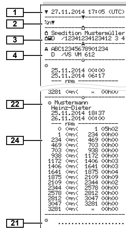
Распечатка профилей частоты вращения
