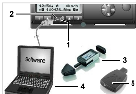
Рис. 51. Подключение к тахографу через интерфейсный разъем
