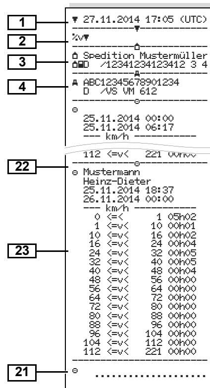
Распечатка профилей скорости
